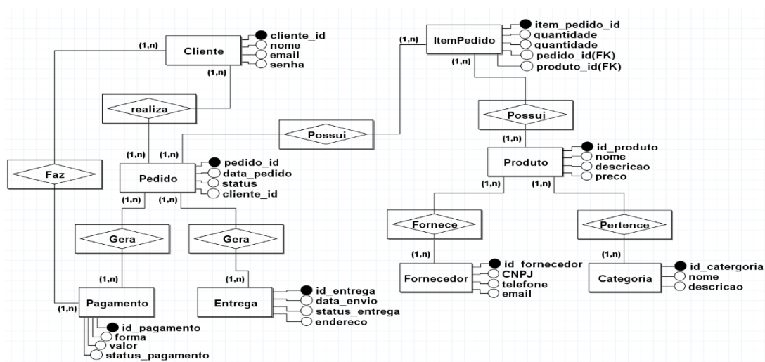
Figura 1. Diagrama de Entidade e Relacionamento (DER)
